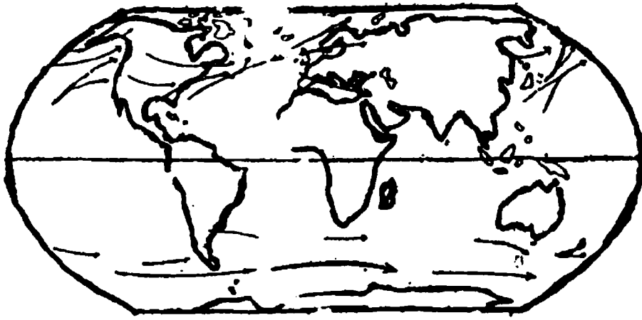
مسارات أعاصير العروض الوسطى
